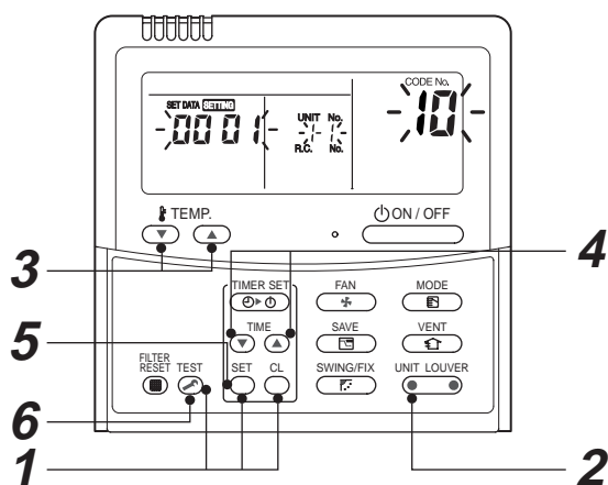
<Fig. 1 RBC-AMT32E>
