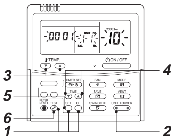
<Fig. 2 RBC-AMS41E>
