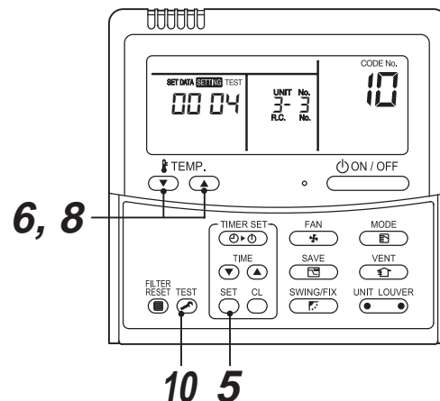
<Fig. 1 RBC-AMT32E>
