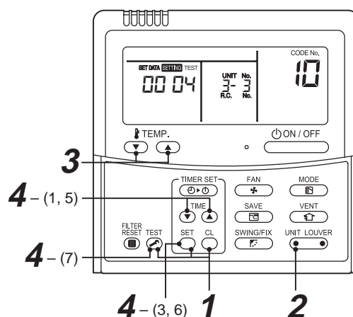
<Fig. 1 RBC-AMT32E>
